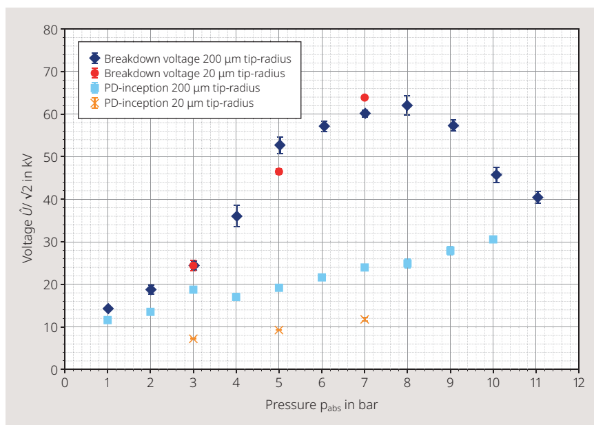
Bild 4 Je höher der Druck, desto näher kommen sich die TE-Einsetzspannung und die Durchbruchspannung (Medium synthetische Luft).
