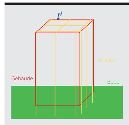
Bild 1 Darstellung der Situation beim Vergleich der Berechnungsmethoden für den Trennungsabstand.
