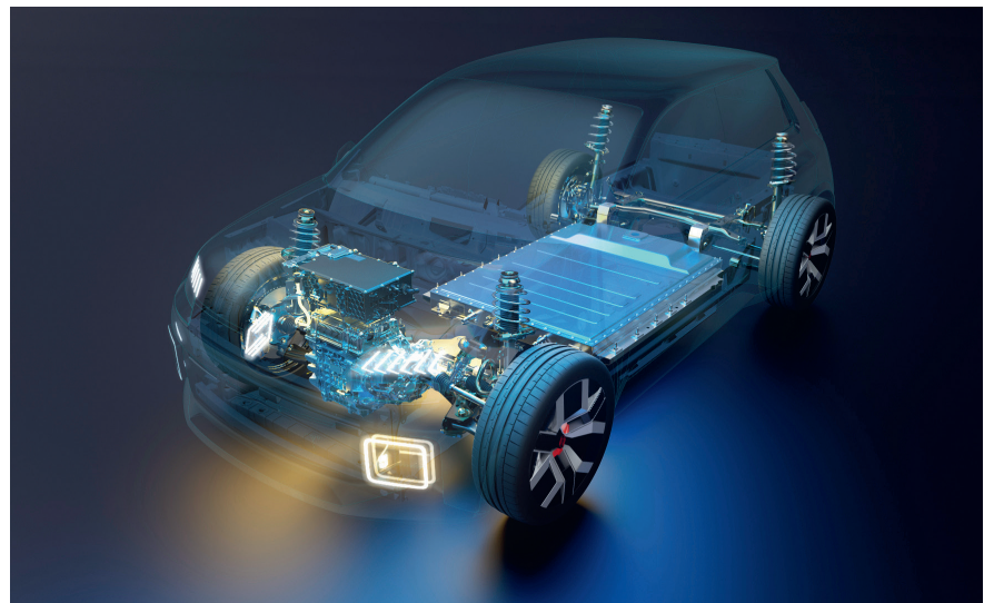
Figure 2 La Renault 5 sera la première voiture électrique de la marque à être dotée d'un chargeur bidirectionnel embarqué. Elle sera commercialisée avec la fonctionnalité V2G en 2024.
