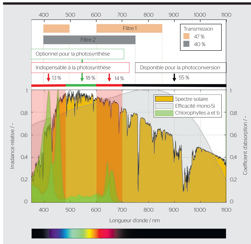
Figure 3 Spectre solaire AM1,5, parties du spectre utilisées par les chlorophylles des plantes [2] et bandes de transmission des deux types de filtres testés. Au-dessus de 700 nm, l'énergie solaire n'est pas utilisée par les chlorophylles et est donc disponible pour la photoconversion dans les panneaux solaires. L'efficacité de conversion photovoltaïque du silicium monocristallin [3] montre l'importance des infrarouges pour la production énergétique.
