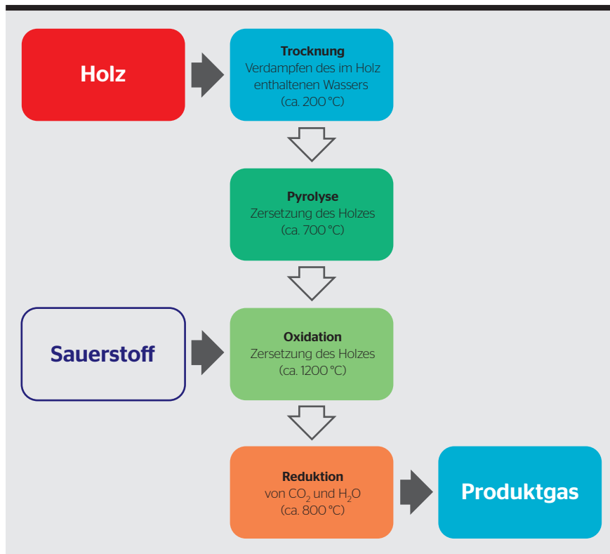
Bild 1 Die vier Phasen der Holzvergasung.
