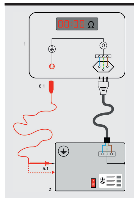
Bild 3 Skizze D.4.3 zur Messung des Schutzleiterwiderstandes.
