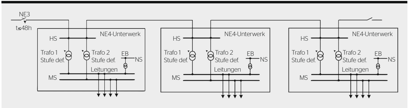
Bild 5 Prinzipschema Beispiel Zuschaltung von drei Unterwerken ab einem Stützpunktunterwerk.
