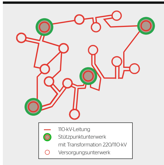
Bild 2 Ausschnitt Axpo-Verteilnetz mit Stützpunkt- und Versorgungsunterwerken.
