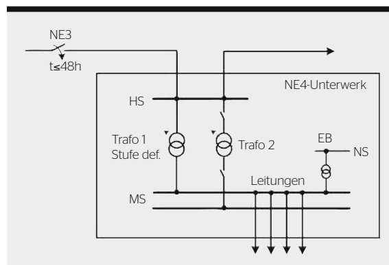
Bild 3 Prinzipschema Ausgangszustand im Versorgungsunterwerk.
