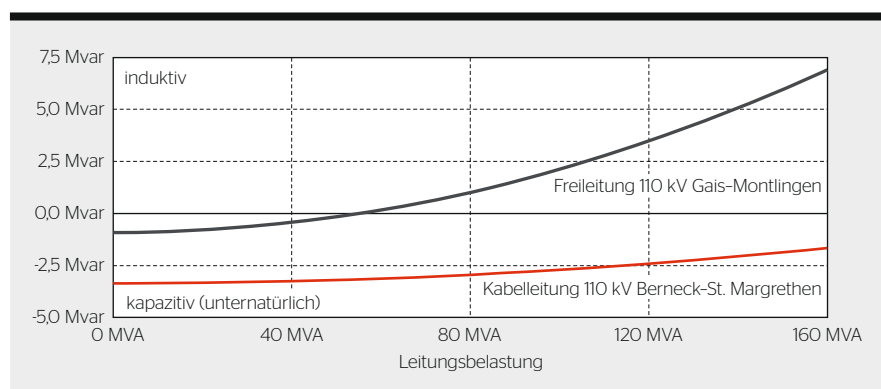
Bild 4 Blindleistungsverhalten einer Frei- und einer Kabelleitung.
