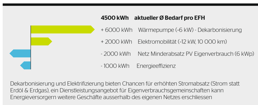
Bild 2 Veränderungen des Energie- und Leistungsbedarfs von Haushaltskunden.
