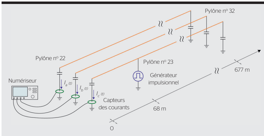
Figure 4 Représentation schématique de la configuration expérimentale. Le second circuit triphasé (non représenté sur ce schéma) était en circuit ouvert aux deux extrémités.
