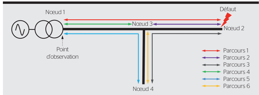
Figure 1 Chemins couverts par les ondes transitoires générées par un défaut apparaissant sur le noeud 2.
