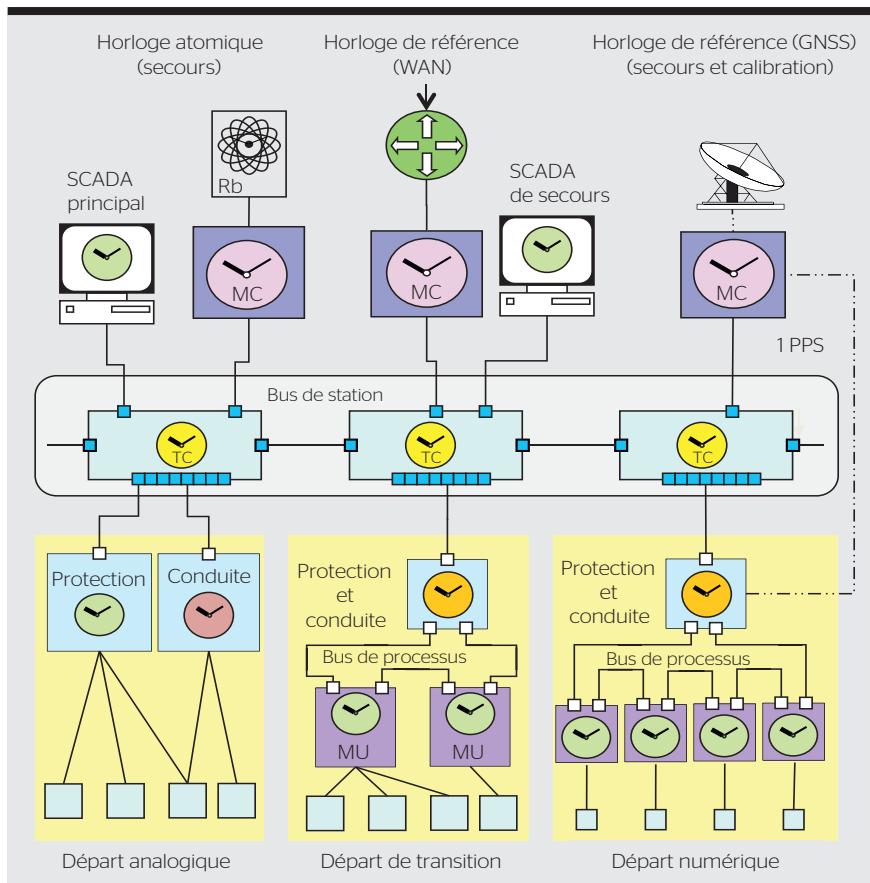
Figure 9 Distribution horaire dans un poste.
