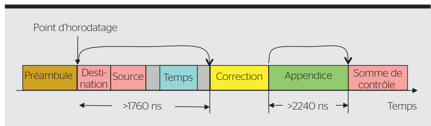
Figure 3 Message Sync dans PTP.
