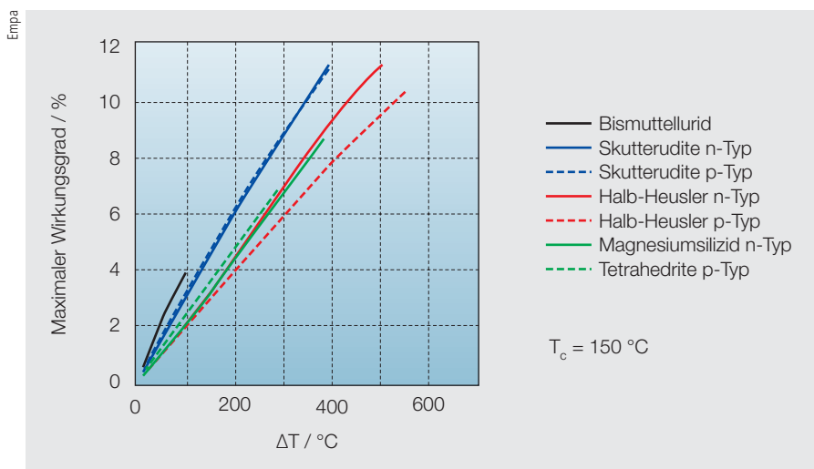
Wirkungsgrade in Abhängigkeit der Temperaturdifferenz für verschiedene Materialien.
