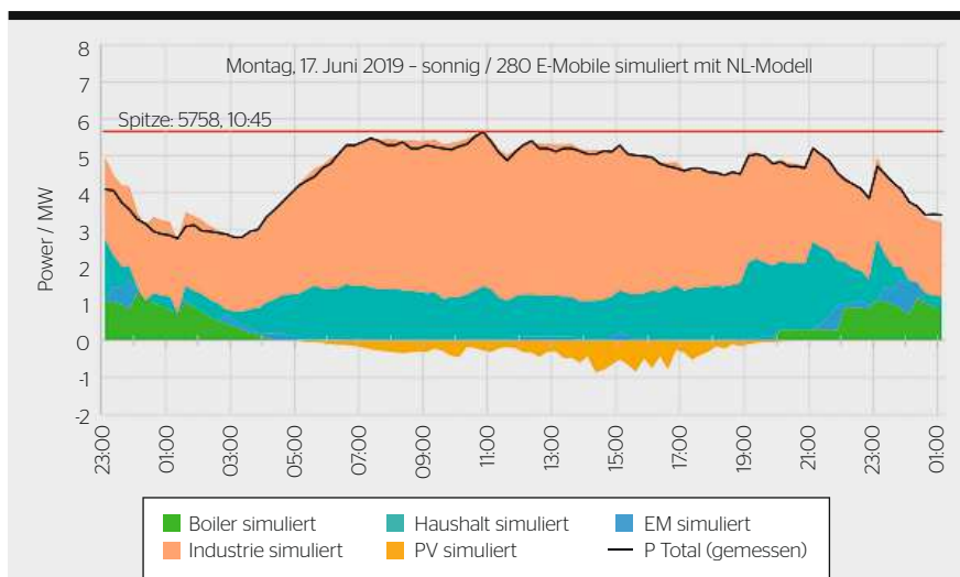
Bild 2 Der berechnete Lastgang aus dem Energiemodell stimmt gut überein mit dem effektiven Verbrauch der Gemeinde Fehraltorf (schwarze Kurve).
