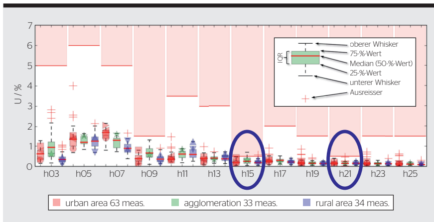
Bild 3 Box-Whisker-Plott, Mess- und Grenzwerte Spannungsharmonische. [1]
