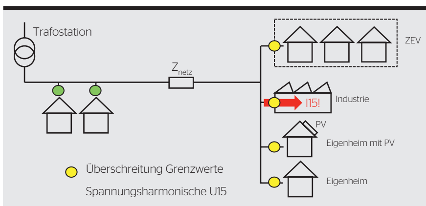
Bild 4 Problemsituation und Analysemöglichkeit der harmonischen Oberwellen.
