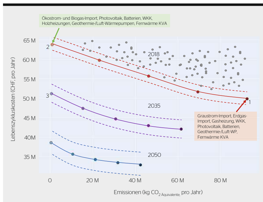
Bild 6 Pareto-Fronten der Energieversorgung der Stadt Chur für die Jahre 2018, 2035 und 2050. Graue Punkte zeigen mögliche Lösungen für 2018, welche jedoch nicht optimal sind. Farbige sind die optimalen Lösungen, die Pareto-Fronten und deren Unsicherheiten (gestrichelte Linien) dargestellt. Pareto-Punkt 1 zeigt die kosten-minimale Lösung und Pareto-Punkt 2 zeigt die nachhaltigsten Lösungen für 2018. Pareto-Punkt 3 zeigt die nachhaltigste Lösung (Netto-null-Szenario) 2035, welche in etwa die gleichen Kosten verursacht wie die Ist-Situation 2018.
