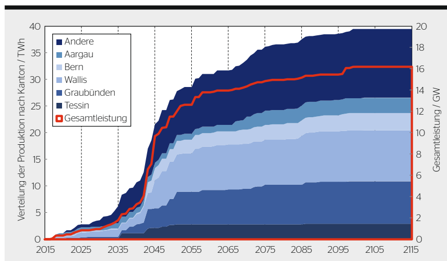
Bild 1 Entwicklung Konzessionsende von Wasserkraftanlagen in der Schweiz.
