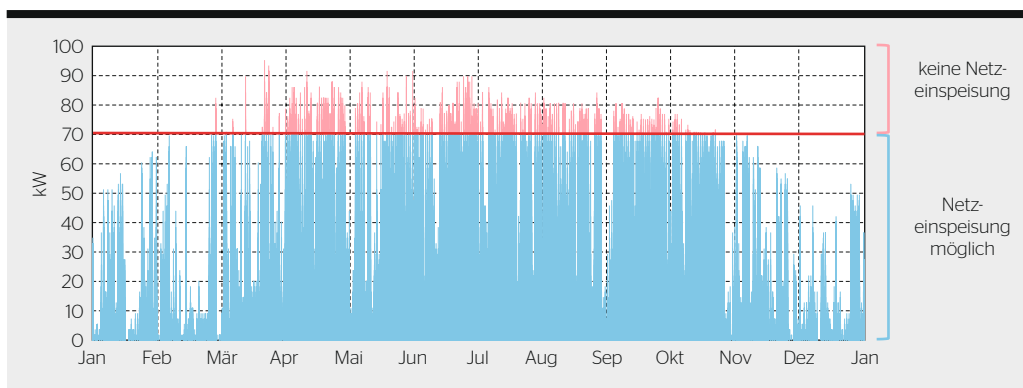
Bild 1 Limitierung bei 70 % der maximalen PV-Panel-Peak-Leistung (Beispiel-Anlage).
