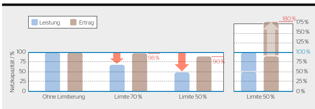
Bild 3 Mehrertrag gesamtheitlich bei gegebener Netzkapazität.
