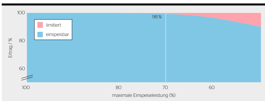
Bild 2 Einspeisbare Produktionsmenge in Abhängigkeit der maximalen Einspeiseleistung (Beispiel-Anlage).
