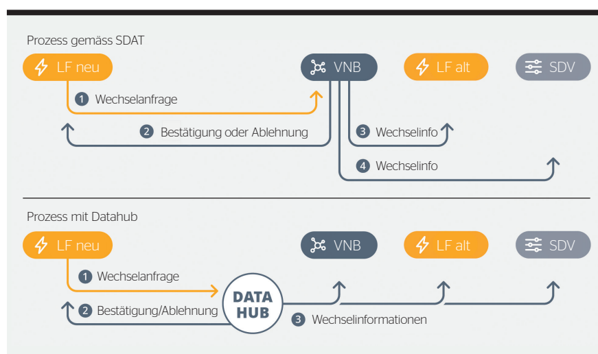
Bild 2 Ergänzend zur Routing-Funktionalität führt der Swisselindex Datahub auch ein Messpunktregister, das mittels Shortcuts für den Netzbetreiber eine vereinfachte Abwicklung der Wechselprozesse ermöglicht.
