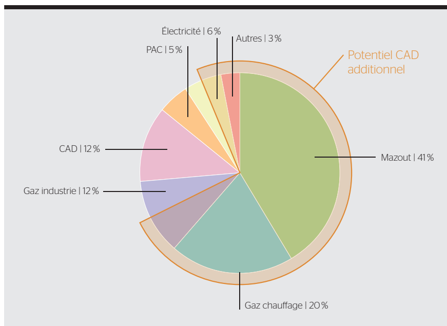
Figure 1 Le potentiel du remplacement des vecteurs énergétiques d'origine fossile par des vecteurs renouvelables dépasse 60 %.
