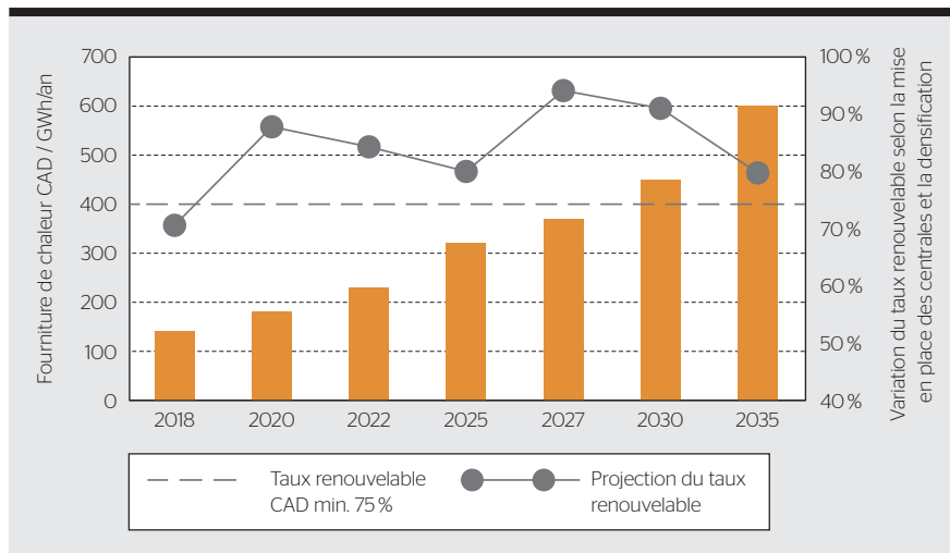
Figure 2 Projection de la fourniture de chaleur via le réseau de chauffage à distance Fribourg à l'horizon 2035. Une croissance des raccordements de 20 à 30 GWh/an est envisageable.
