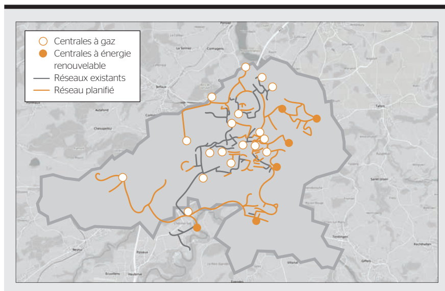
Figure 3 La mise en réseau de tous ces noyaux est en cours et représente un point-clé de la stratégie de Groupe E Celsius.
