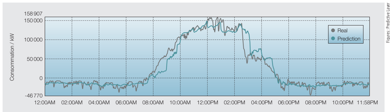
Figure 4 Modèle prévoyant la consommation d'énergie électrique d'une ville quotidiennement.
