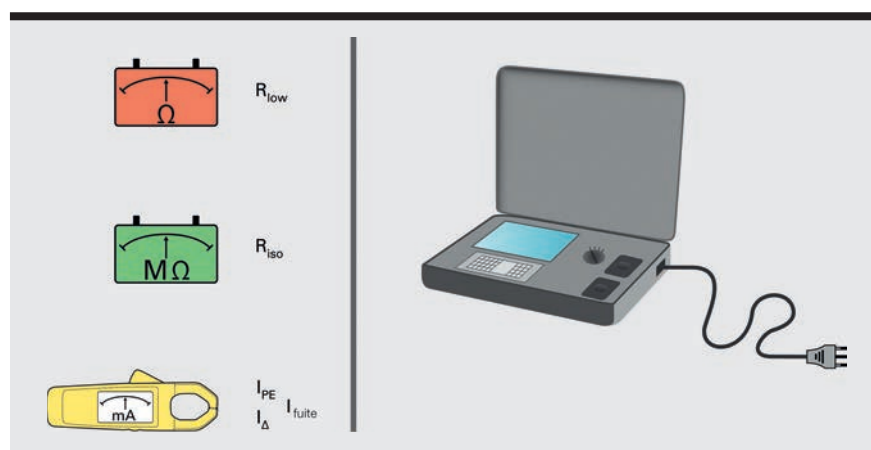
Figure 2 Les mesures peuvent être réalisées avec des appareils de mesure individuels ou des testeurs d'appareils.
