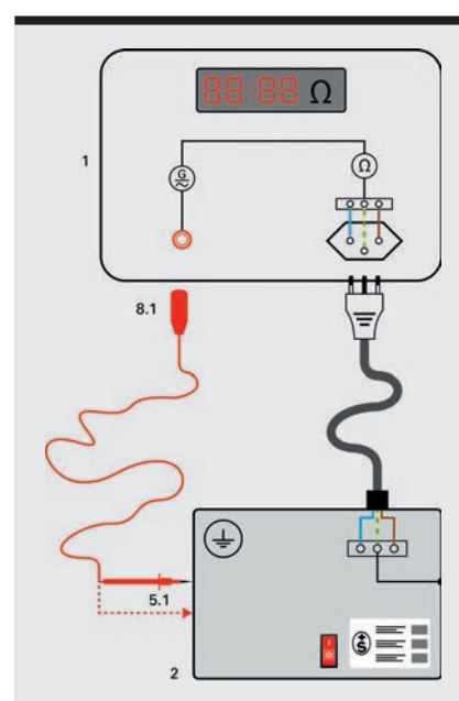
Figure 3 Schéma D.4.3 pour la mesure de la résistance du conducteur de protection.
