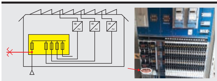
Figura 3 Esempio 3: Impianto fotovoltaico con stazione di trasformazione privata.
