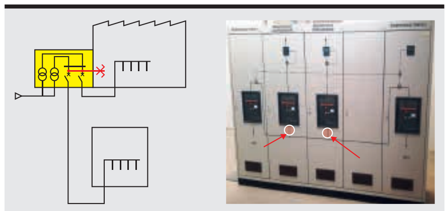
Figura 2 Esempio 2: Stazione di trasformazione privata in ambito industriale e commerciale.
