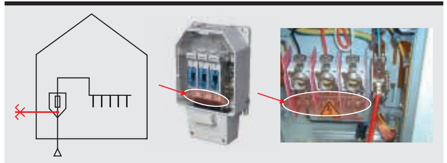
Figura 1 «Caso normale»: ruttore di sovrintensità, 1 cassetta di allacciamento dell'edificio.
