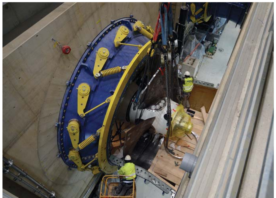
Bild 3 Einbau einer horizontalachsigen Kaplan-Rohrturbine.
