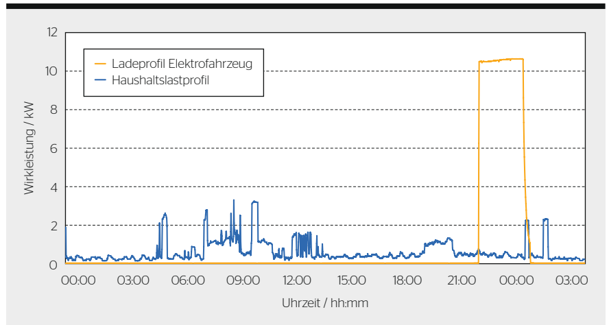
Bild 1 Gängiges Lastprofil mit und ohne Elektrofahrzeug bei einem Einfamilienhaus (Referenzbeispiel mit Ladeleistung 11 kW).
